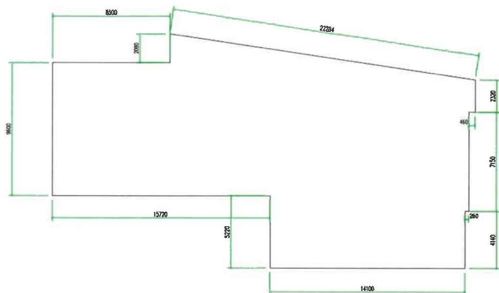
西华路 4 号首层仓库平面图
