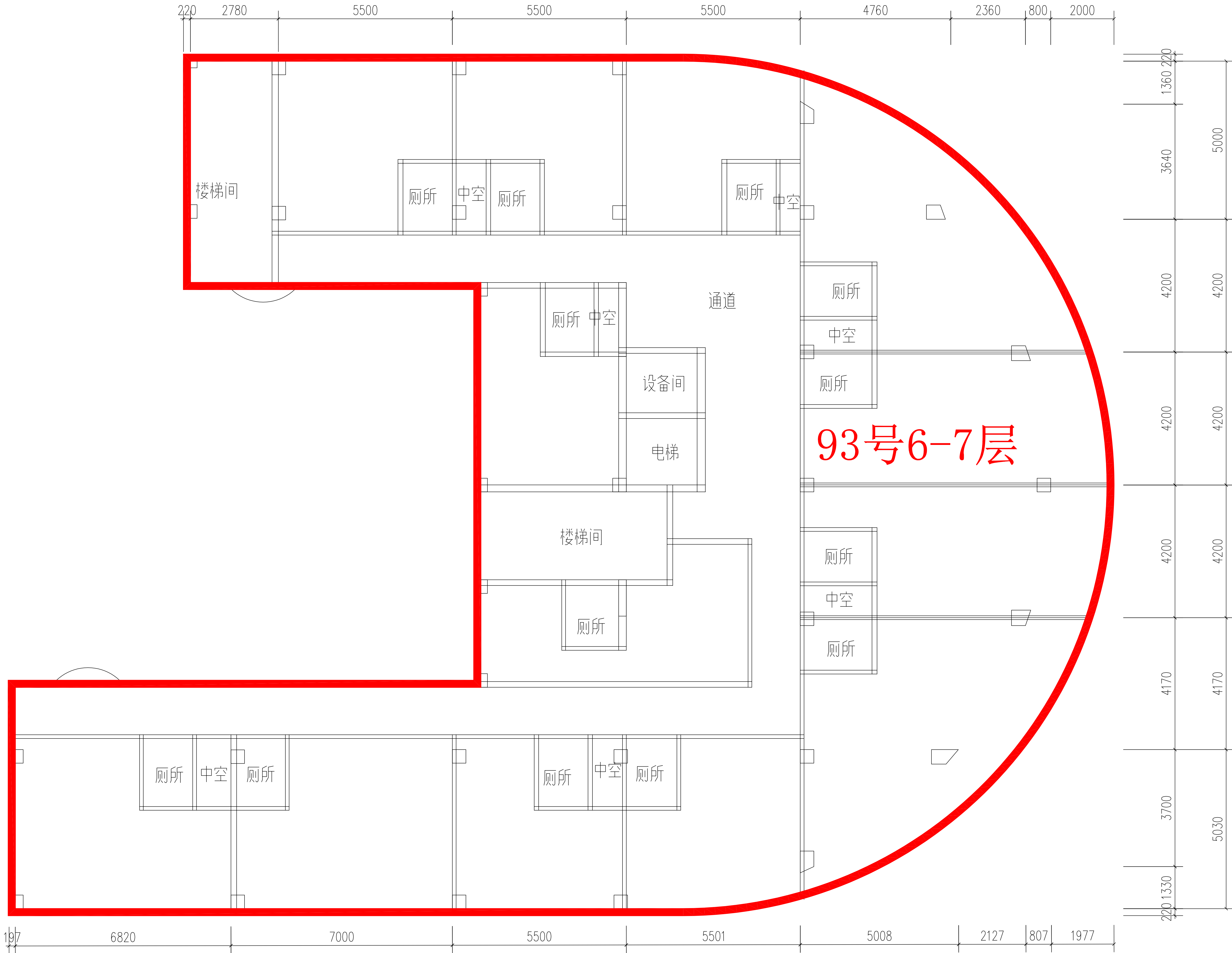
93号6-7层平面图
