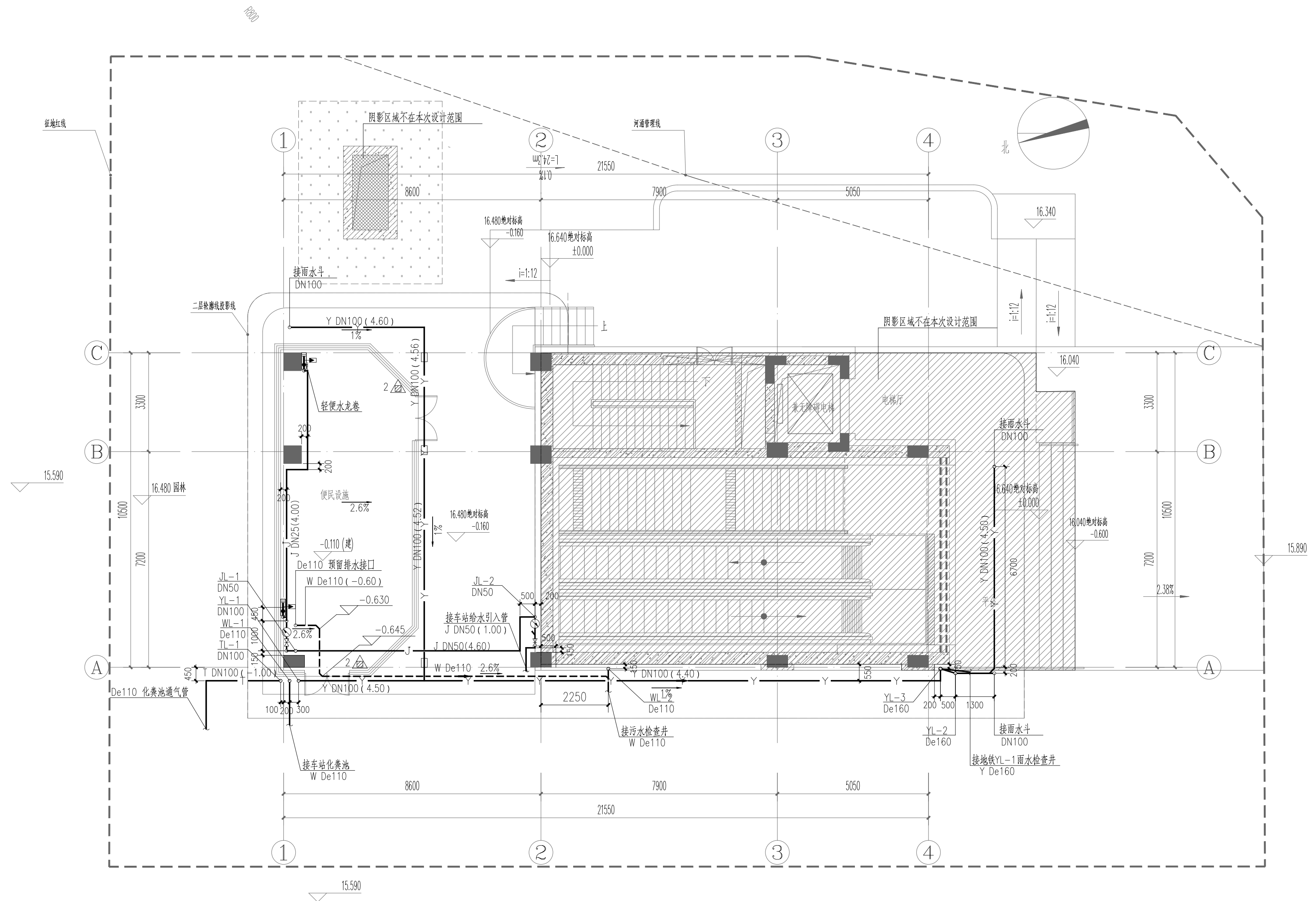
地面便民设施首层给排水及消防平面图 1:100
