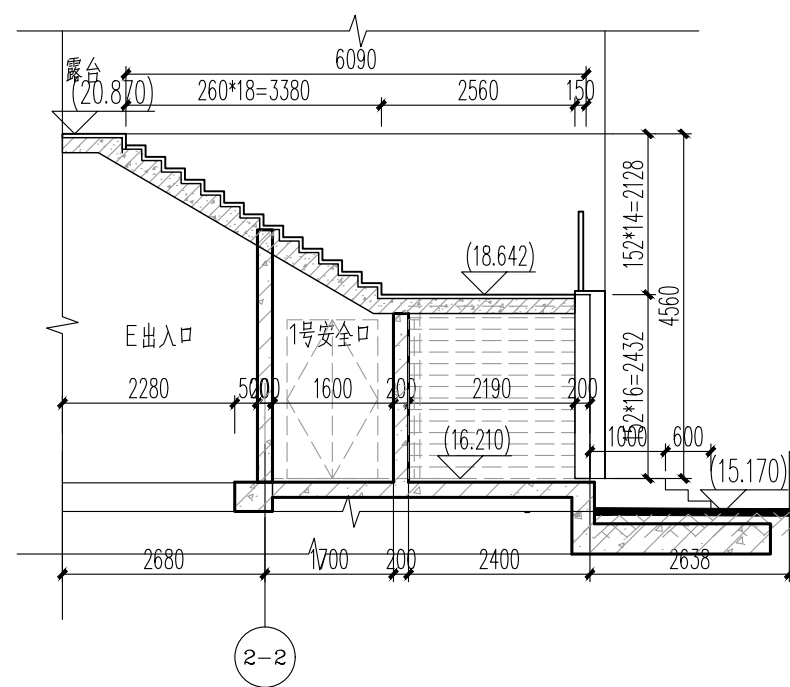
1 室外楼梯2剖面图 1:100
