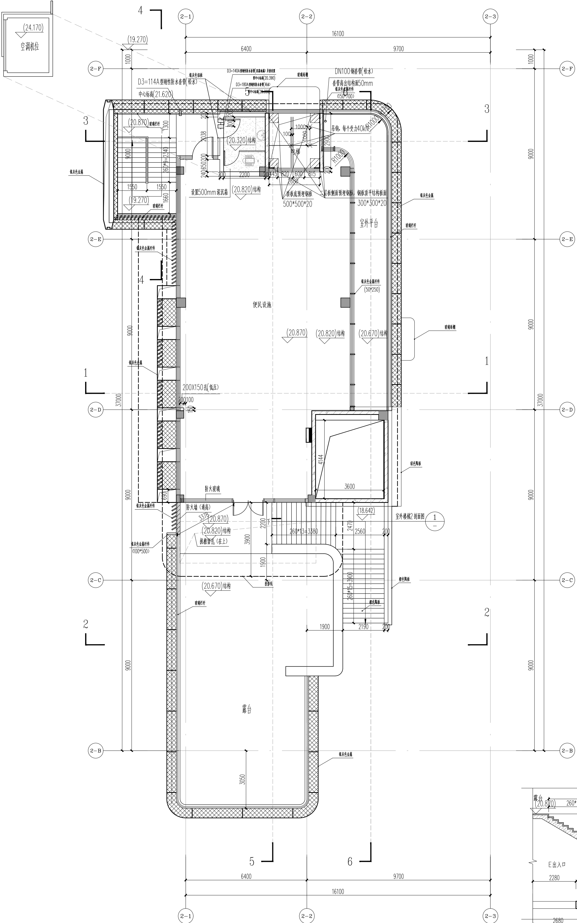
二层平面图 1:100
