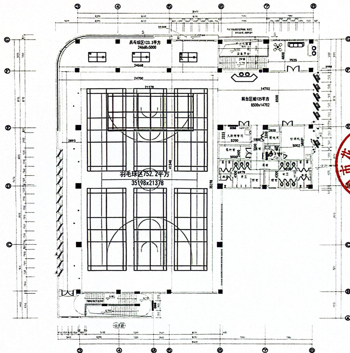
圆玄小学体育馆三层平面图1:100
