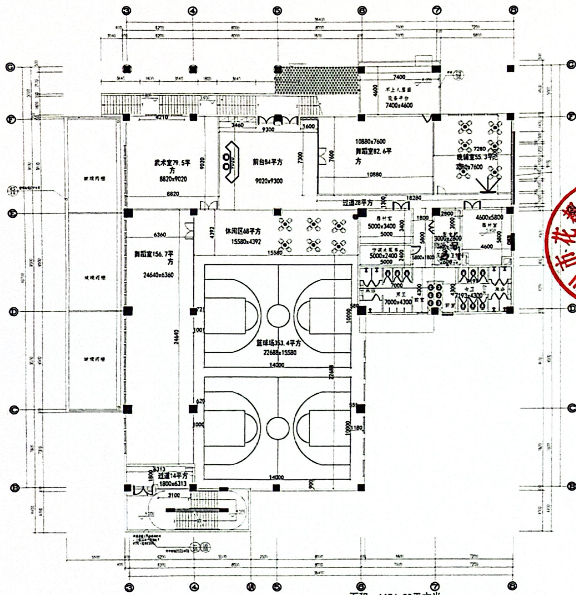
圆玄小学体育馆二层平面图1:100
