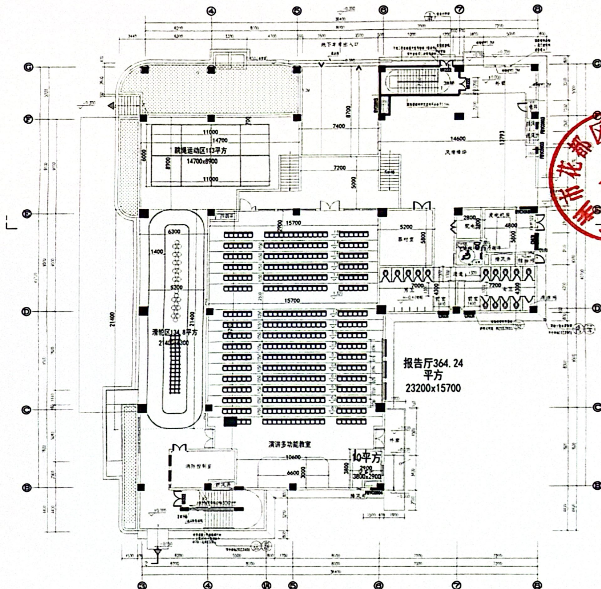
面积: 1399.31平 方米周长: 137 圆玄小学体育馆一层平面图1:100
