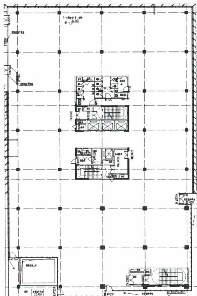
A1 栋 9 层平面图 (2732.62 平方米)
